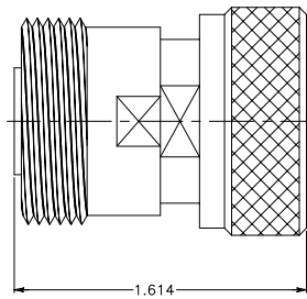
(7/16 Din Plug - 7/16 Din Jack)
